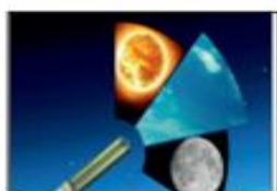
Fig. 1: NASA-AERONET
