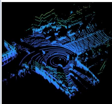
Pandaset_LidarData.tar.gz
