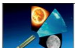
Fig. 1: NASA-AERONET
